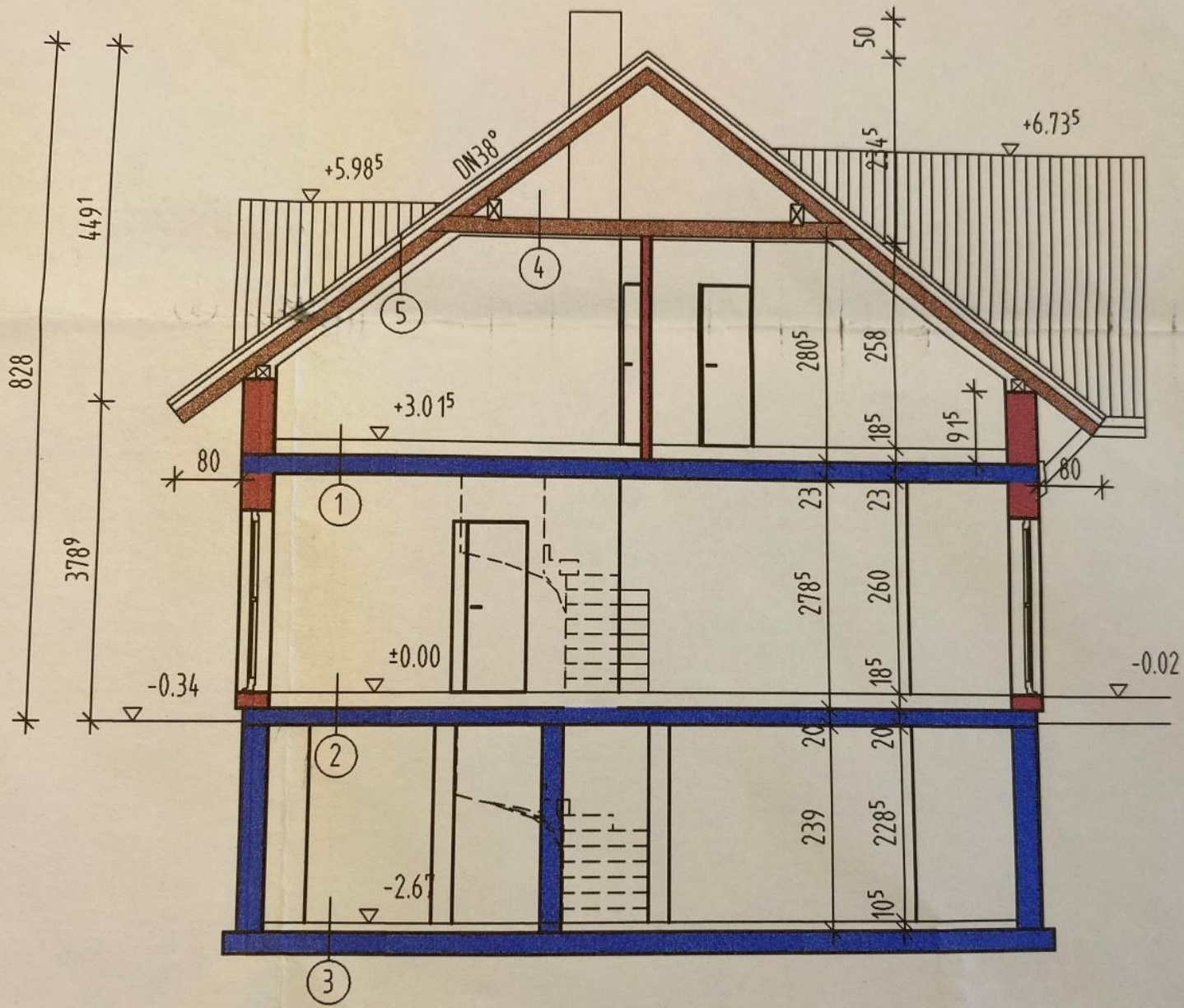
SCHNITT A-A
